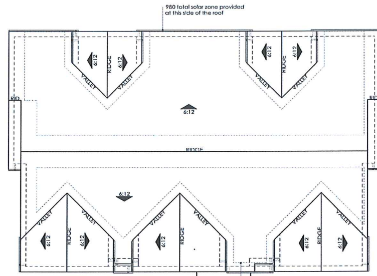
ROOF PLAN OVERHANG : 12" RAISE : 12" ROOF PITCH : 6:12 U.N.O
