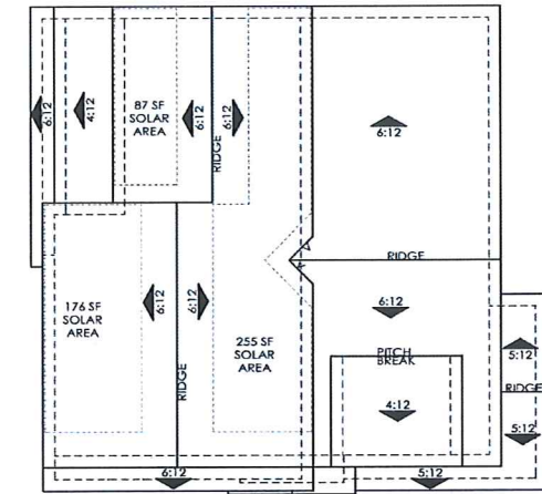
ROOF PLAN OVERHANG: 12" RAKE: 6:12 U.N.O.
